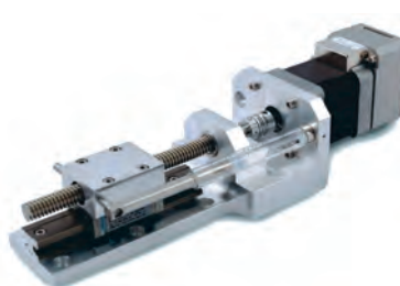
Linear motion
